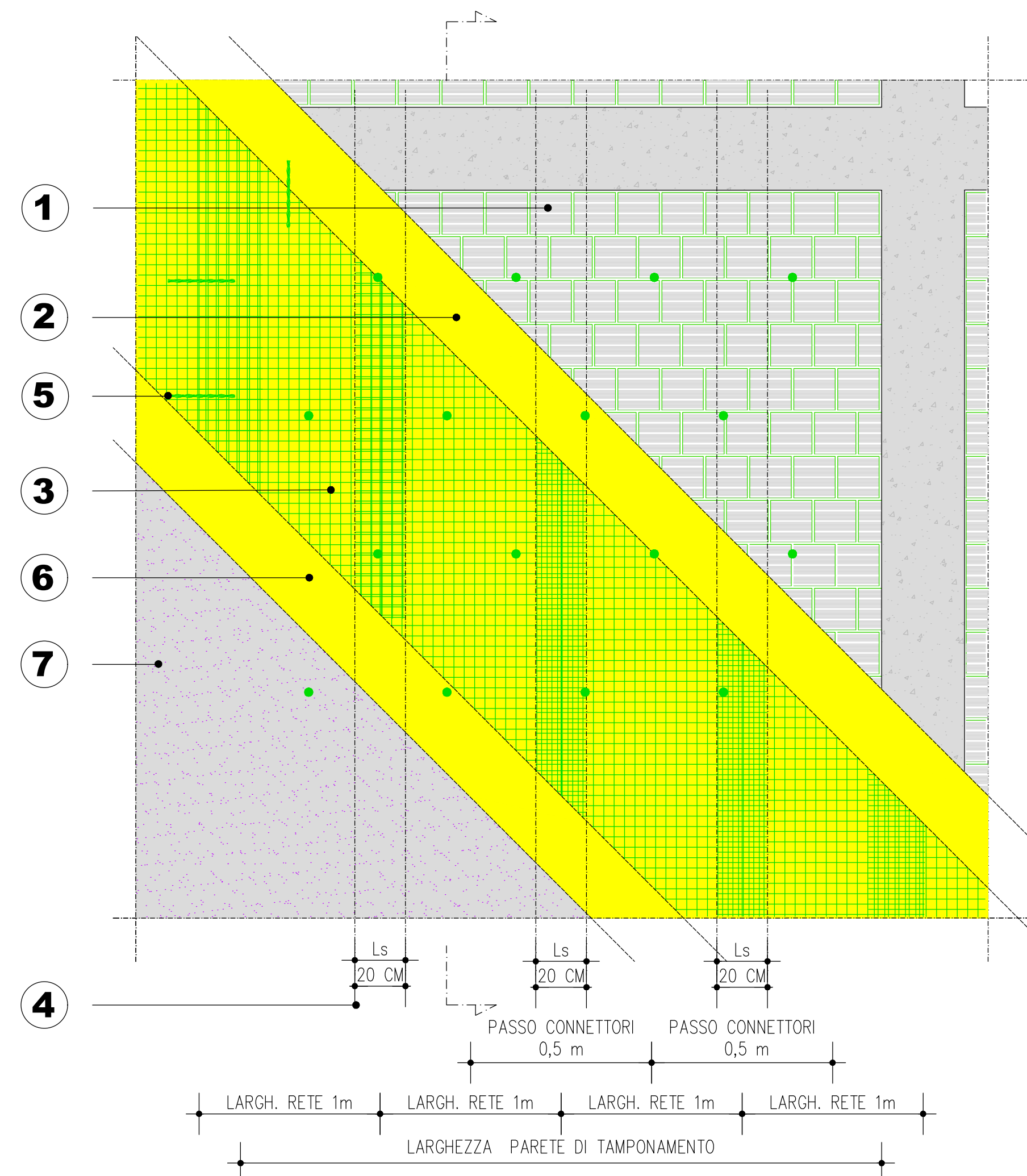
PROSPETTO SISTEMA DI PRESIDIO ANTIRIBALTAMENTO DELLA TAMPONATURA TRAMITE GEO GRID 120 E BARRE STEEL DRYFIX 8
