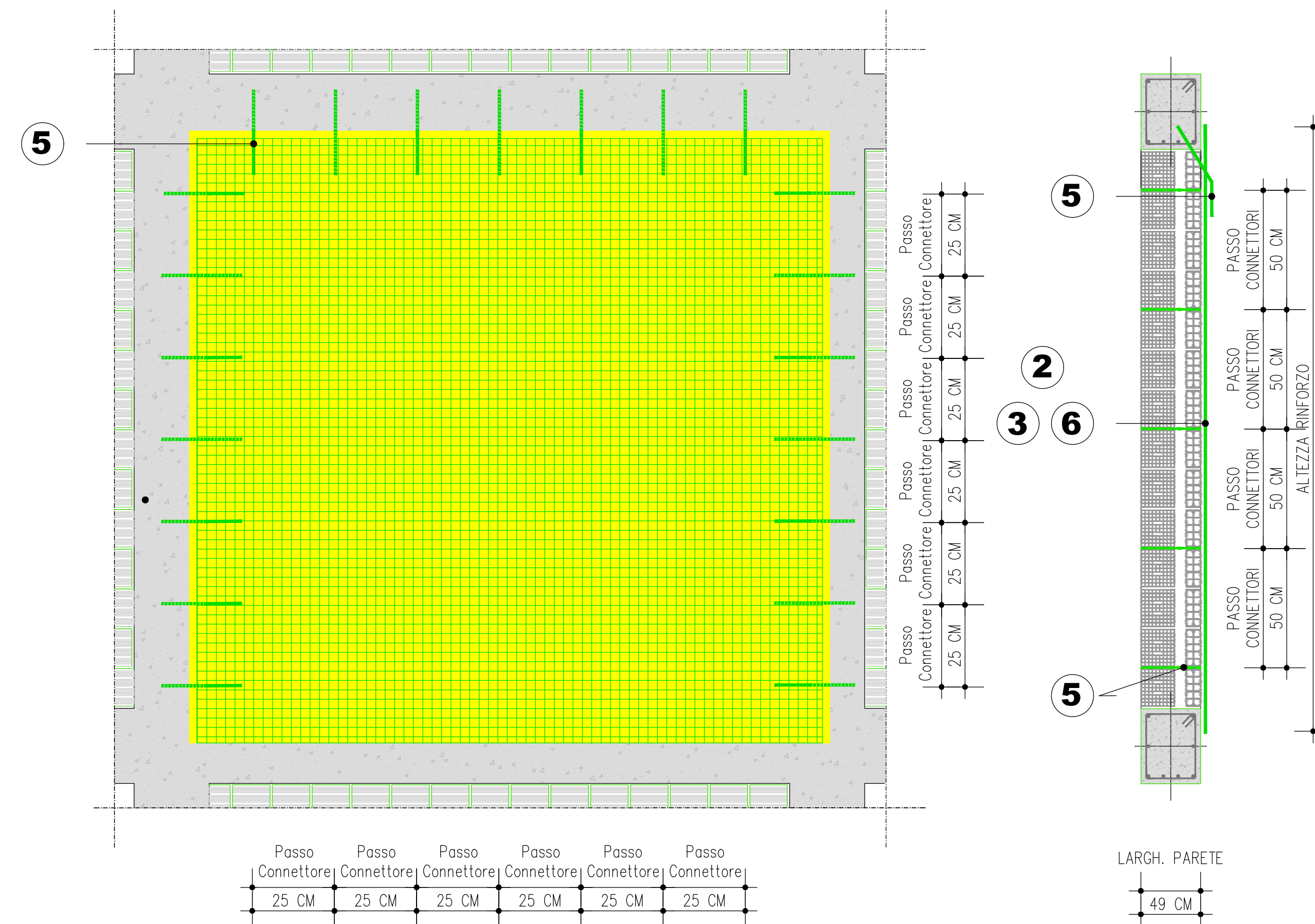
PROSPETTO DI DETTAGLIO E SEZIONE A-A' INSTALLAZIONE A SECCO BARRE STEEL DRYFIX 8 LUNGO LO SVILUPPO DEL TELAIO IN CEMENTO ARMATO E PRESIDIO ANTIRIBALTAMENTO MEDIANTE GEO GRID 120 E BARRE STEEL DRYFIX 8
