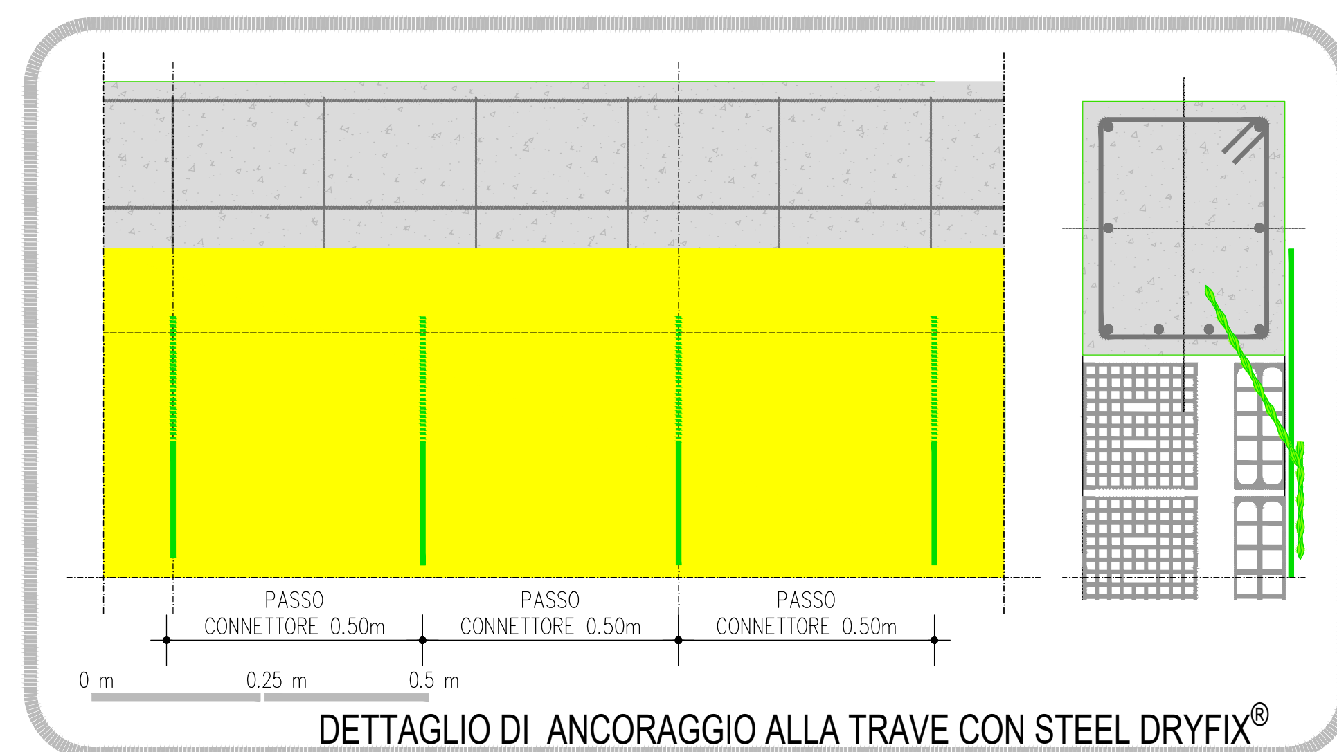
PROSPETTO SISTEMA DI PRESIDIO ANTIRIBALTAMENTO DELLA TAMPONATURA TRAMITE GEO GRID 120 E BARRE STEEL DRYFIX 8
